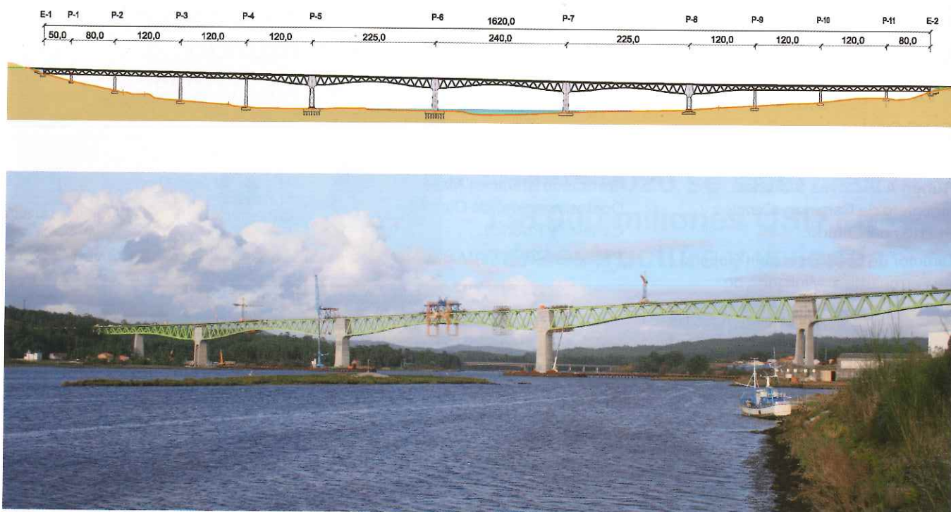
Figs. 1a y 1b. Alzado y vista actual del Viaducto sobre el río Ulla (nov. 2014)
