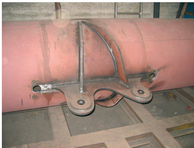
Figura 20. Detalle de las cartelas de unión superior de las péndolas con los tubos de los arcos
