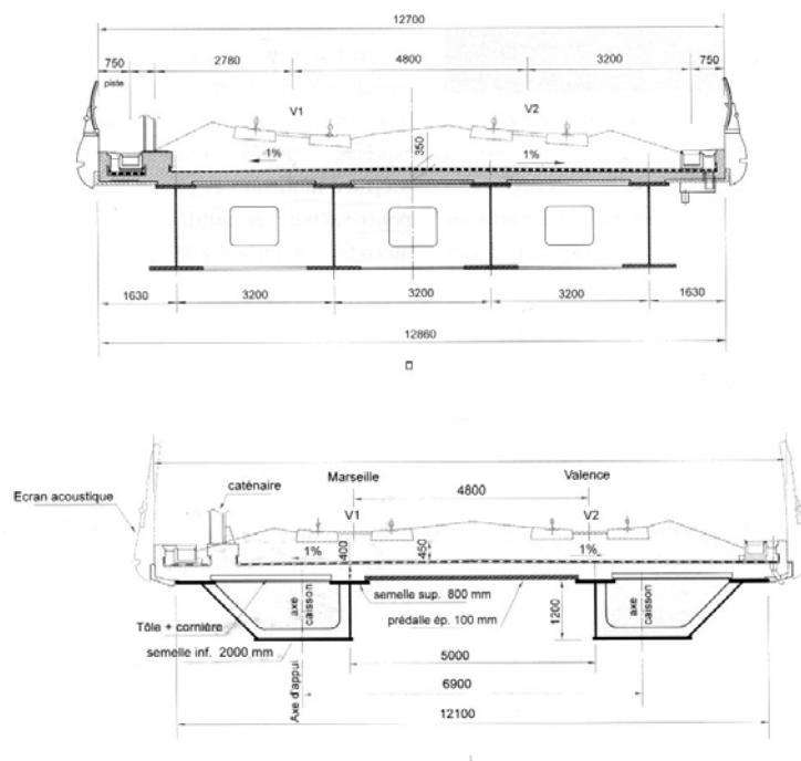
Figura 15. Sección transversal multiviga y con doble cajón
