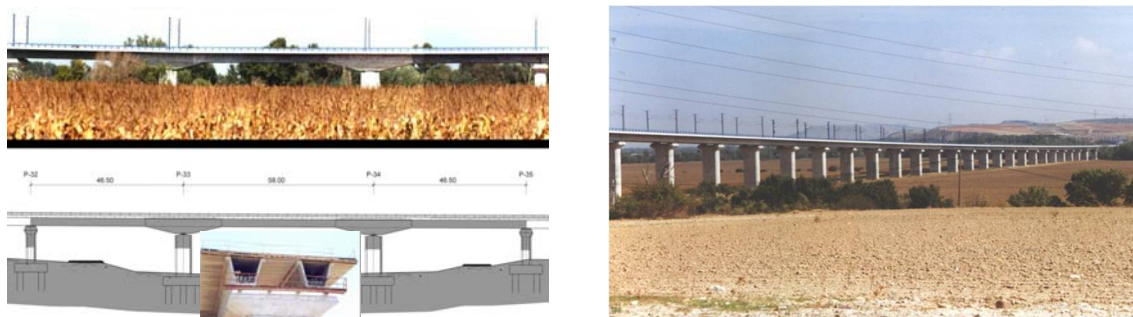
Figura 6. Viaductos prefabricados sobre el Jarama (luz 62m.)
