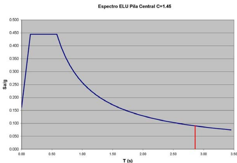
Figura 38. Reducción de la fuerza sísmica por la flexibilidad axil del dintel mixto
