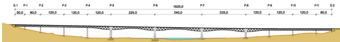
Figura 42. Alzado del Viaducto
