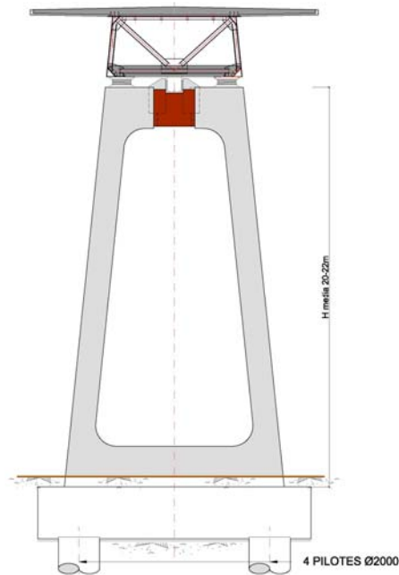
Figura 35. Sección por pila tipo
