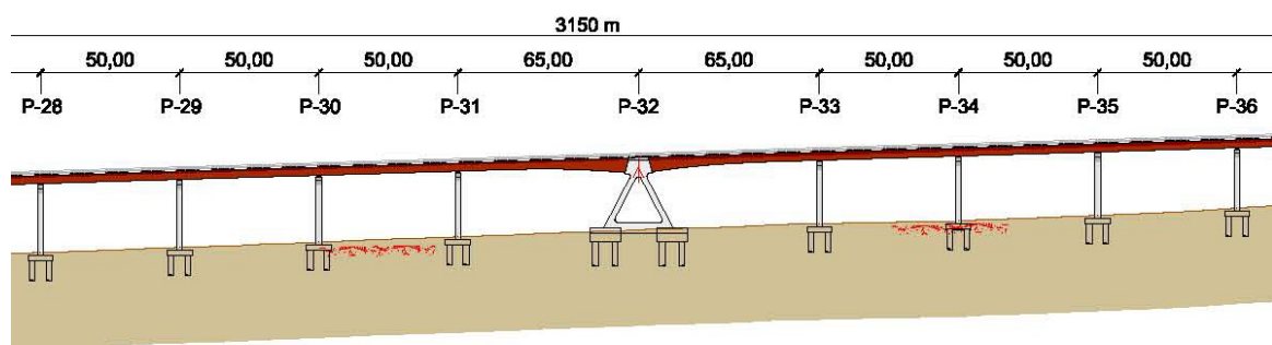
Figura. 36. Alzado del Viaducto
