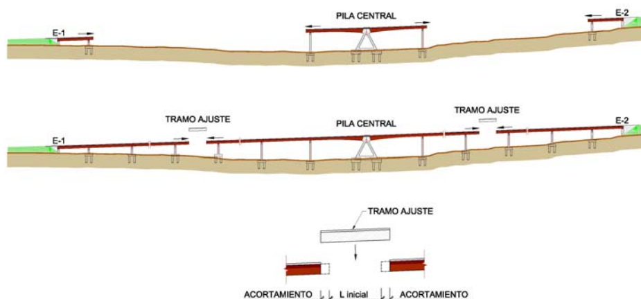
Figura 37. Reducción de la retracción efectiva en la junta por adecuación del proceso constructivo
