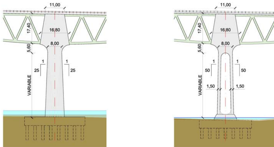
Figura 41. Vista de las pilas centrales (P-6 y P-7) y laterales (P-5 y P-8)
