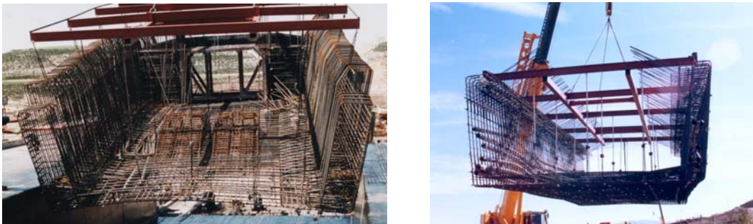
Figura 4. Industrialización de ferralla en montajes con autocimbras
