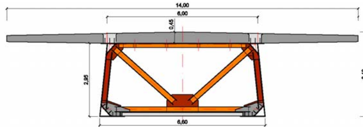
Figura. 34. Sección por centro de vano
