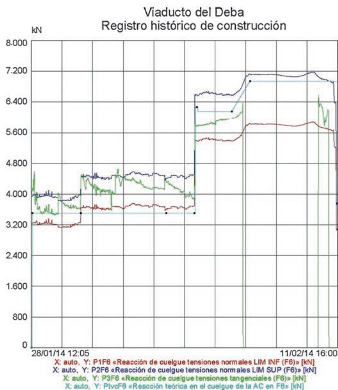
Figura 36. Control de la reacción en el cuelgue de la cimbra autolanzable durante la sexta fase de ejecución del tablero (con una ménsula de 20 m y ejecutada mediante 4 subhormigonados).
