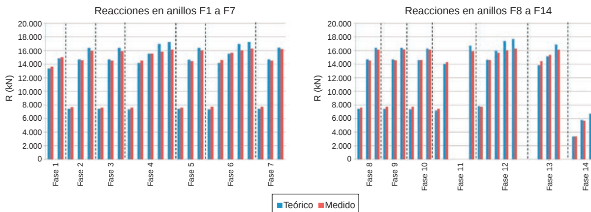
Figura 37. Control de la reacción en el anillo delantero durante las distintas subfases de hormigonado de las 14 fases de ejecución del tablero.
